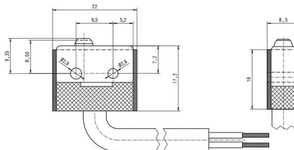
MICROSWITCH DIMENSIONS
